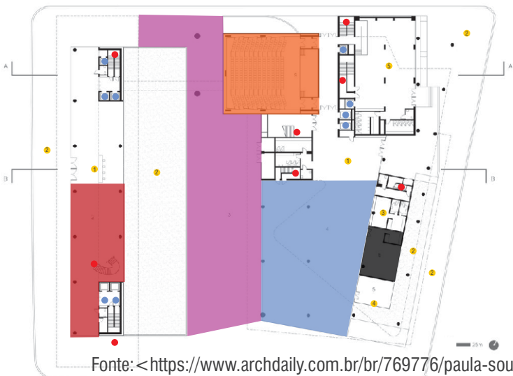
Figura 10. Planta Térrea, Centro Paula Souza.
