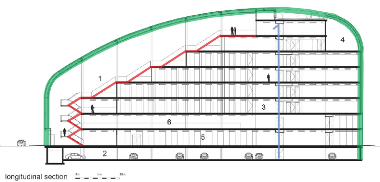
Figura 8. Corte Longitudinal, Análise de Cobertura.
