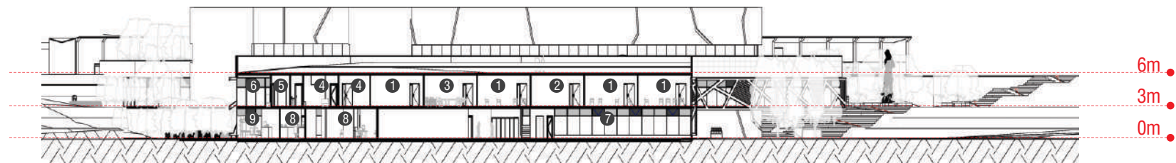
CORTE AA
