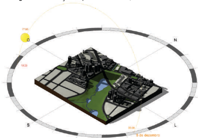
Figura 47. Insolação no período de verão, 2018.
