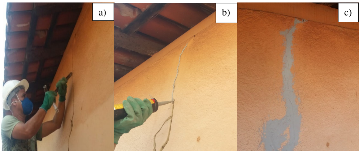
Figura 14. a) preparação do substrato; b) aplicação do selante; c) resultado após aplicação.
