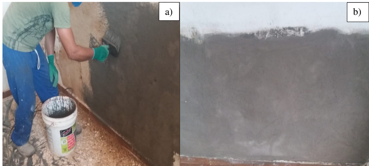
Figura 10. a) aplicação do impermeabilizante; b) resultado após duas demãos.
