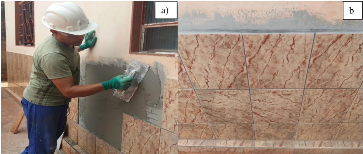
Figura 13. a) aplicação de argamassa para assentamento de revestimento cerâmico; b) revestimento assentado.
