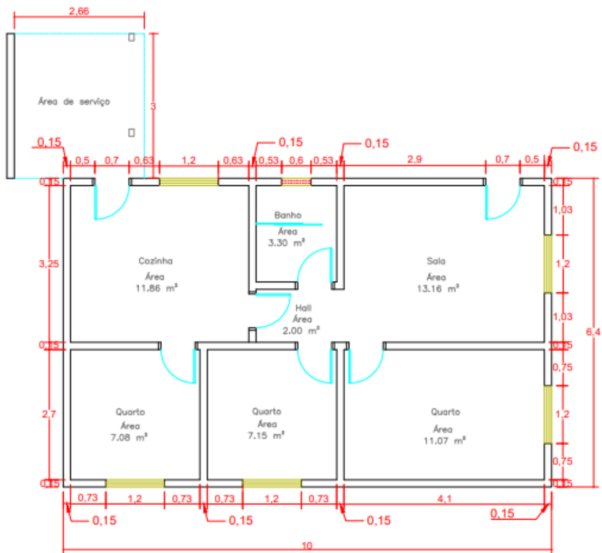
Figura 1. Planta da edificação.
