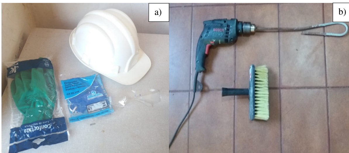
Figura 7. a) epi's utilizados; b) misturador e brocha.
