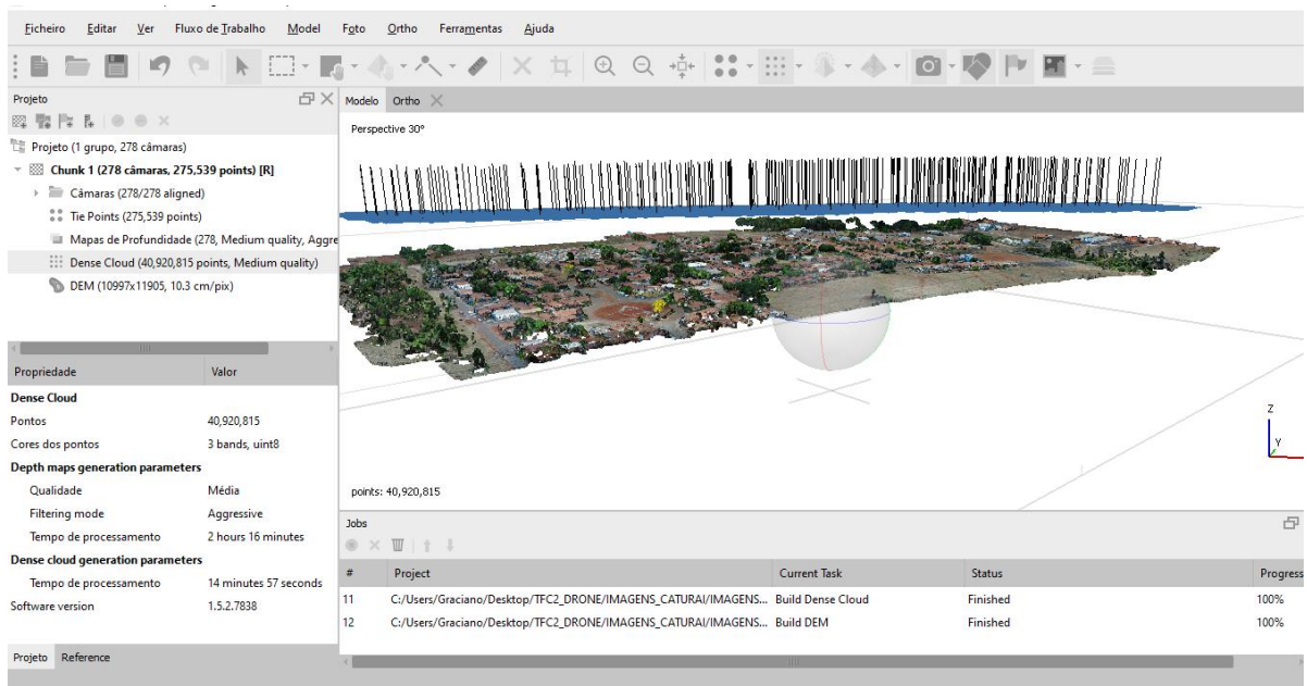
Figura 04 – Alinhamento das fotos e geração da Nuvem Densa de Pontos.
