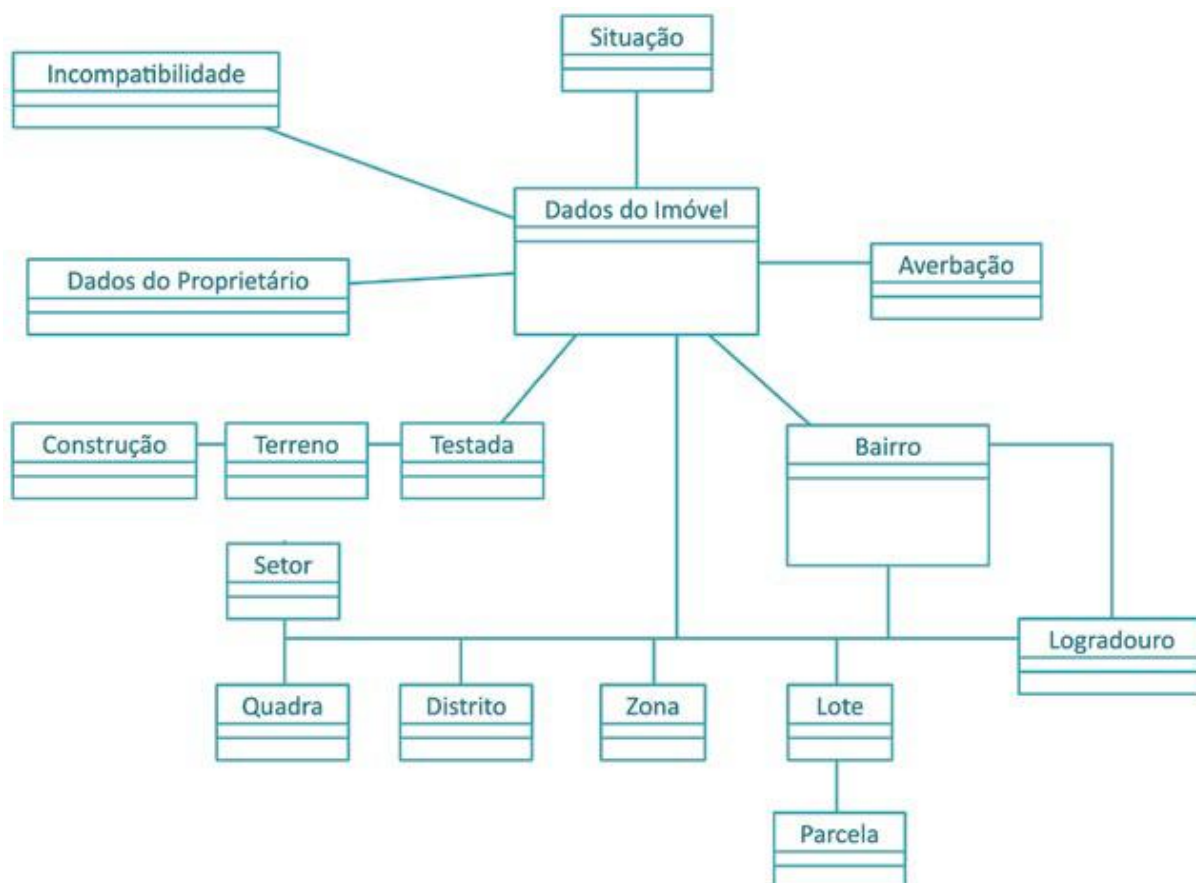
Figura 07. Esquema de um banco de dados cadastral.
