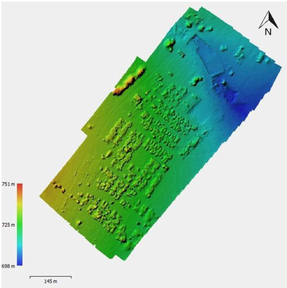
Figura 06 –Modelo Digital de Elevação gerado.
