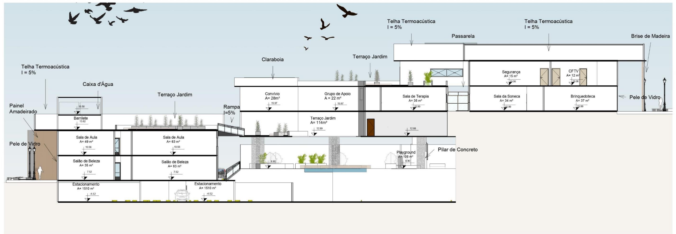
Corte D
