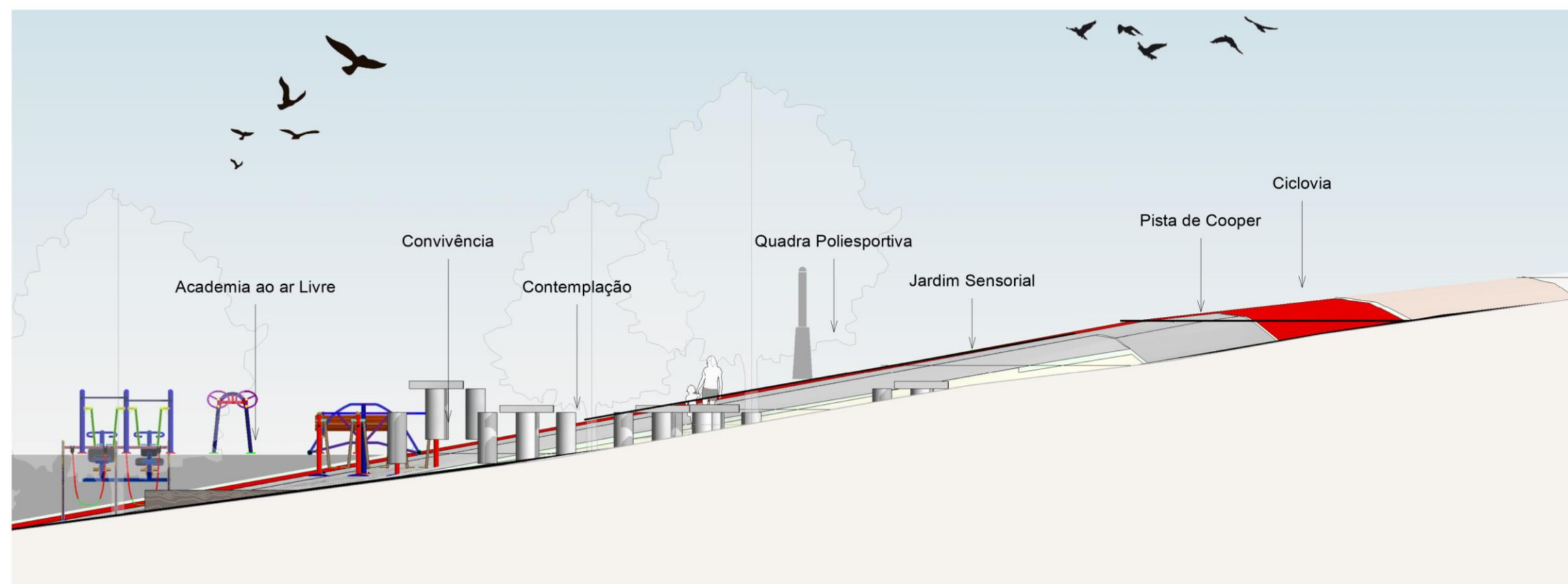
Corte D
