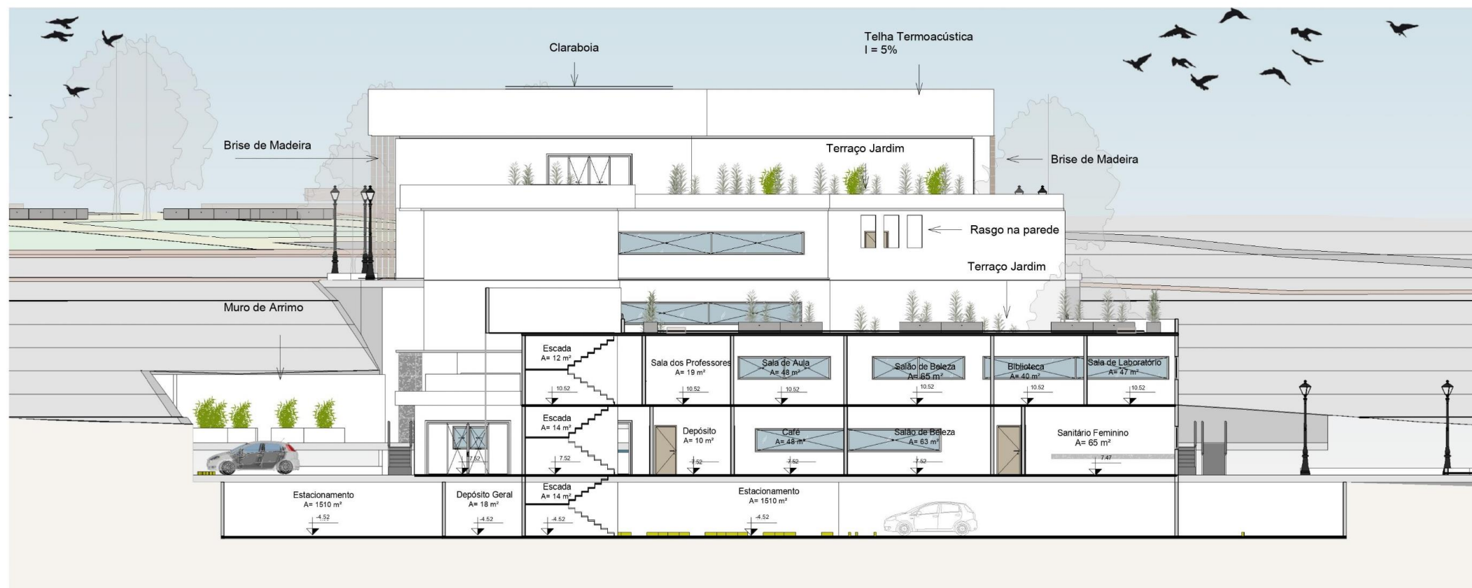
Corte A
