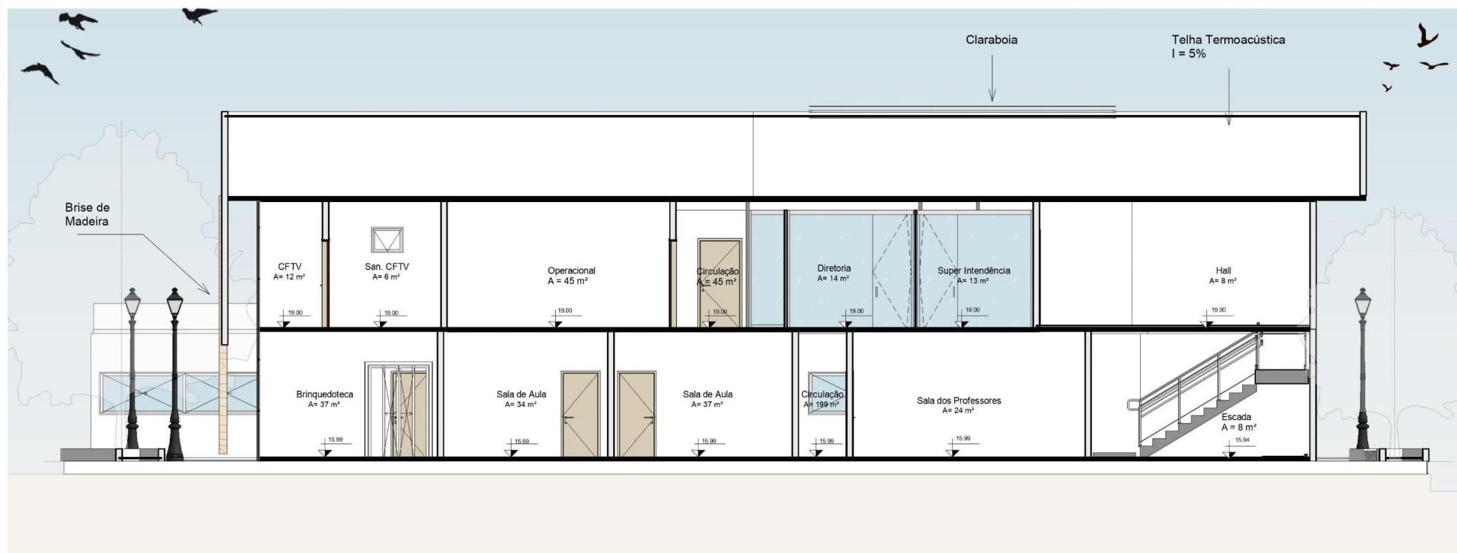
Corte B
