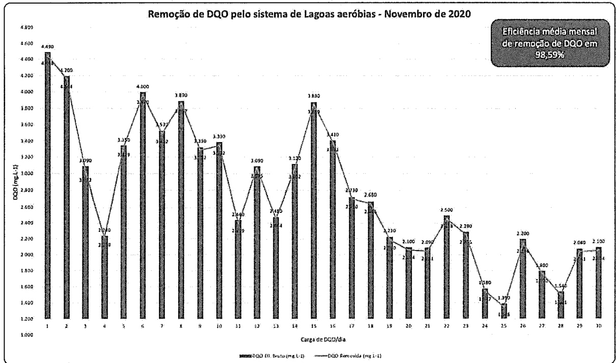
Imagem 03: Gráfico da remoção de DQO em novembro de 2020. Fonte: própria.
