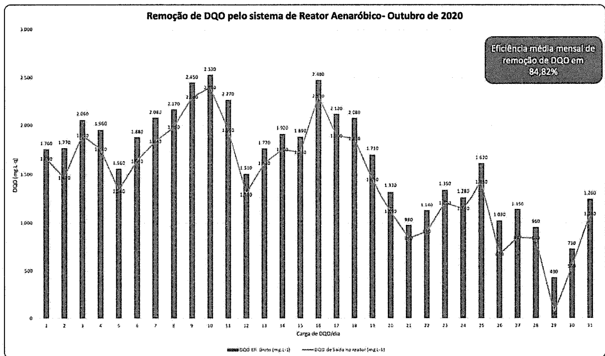
Imagem 06: Gráfico da remoção de DQO no reator anaeróbico em outubro de 2020.
