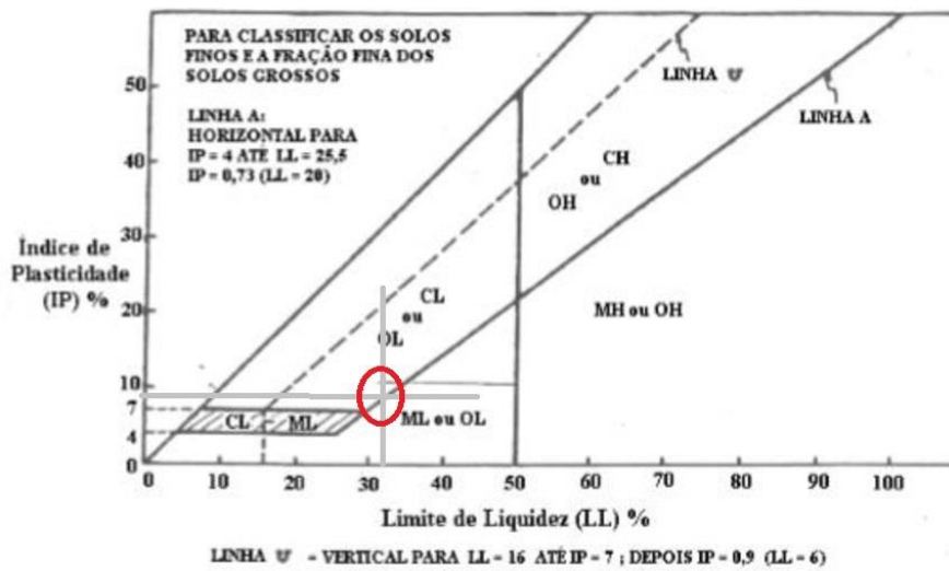
Figura 35. Carta de Plasticidade.
