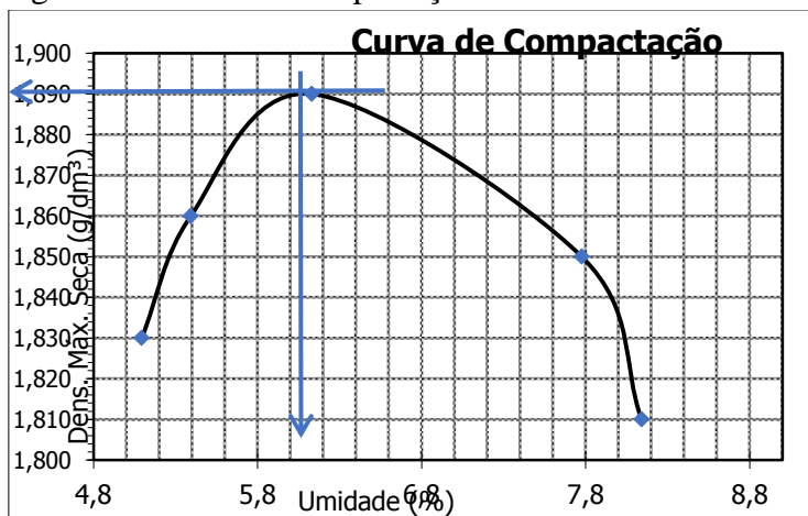
Figura 38. Curva de compactação.
