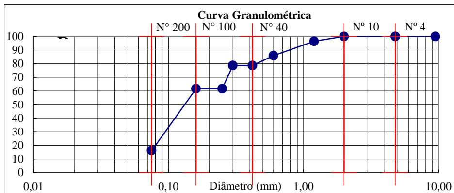
Figura 33. Curva Granulométrica.
