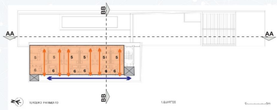
Figura 30: Planta terceiro e quarto pavimento setorizada Fonte: (ALVARENGA, MAIA e ZAMPIERI (2016) Edição: MORAIS, Rhayssa (2018)
