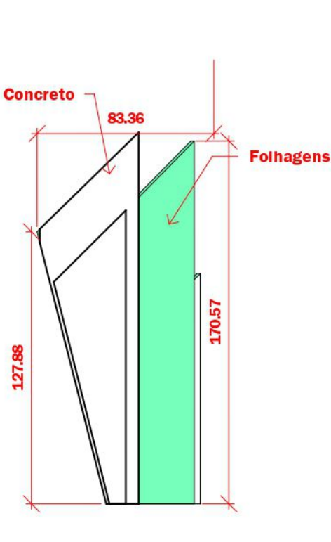
5.4.25.Corte Detalhe 1 - BB Esc: 1/25
