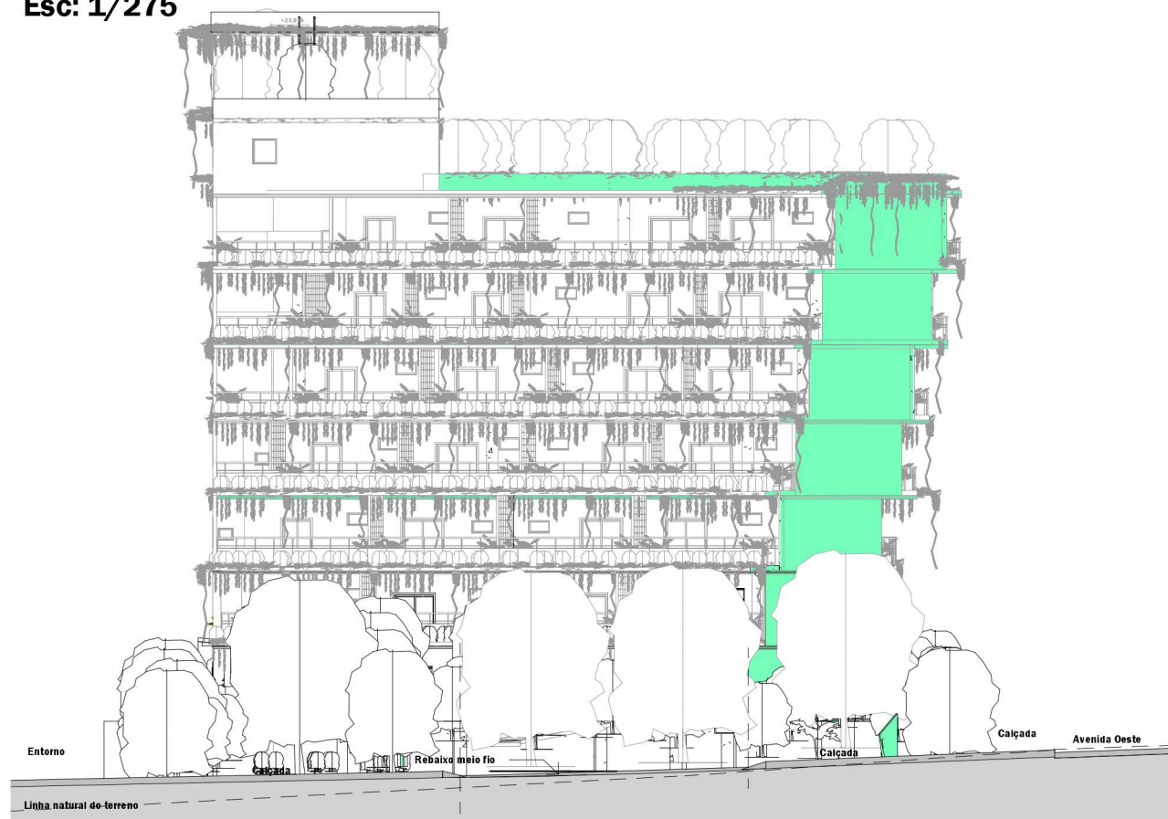
5.4.15.Corte FF
