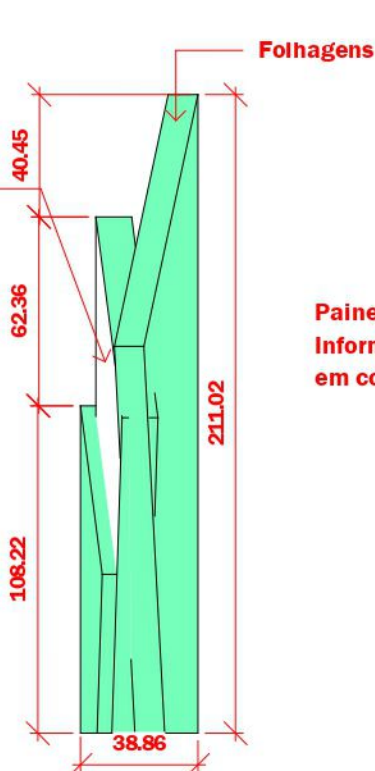
5.4.26. Corte Detalhe 1 - CC Esc: 1/25
