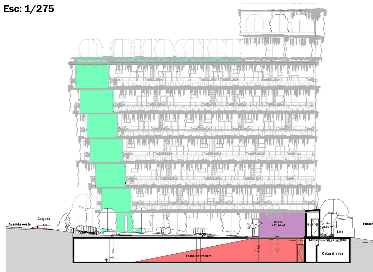
5.4.16.Corte GG
