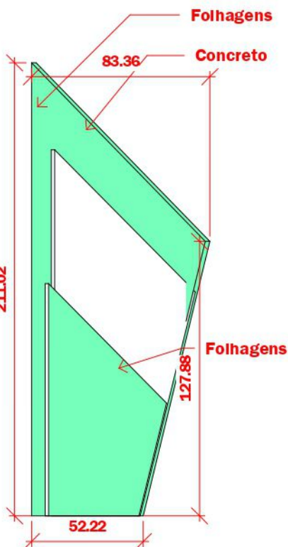
5.4.24.Corte Detalhe 1 - AA Esc: 1/25
