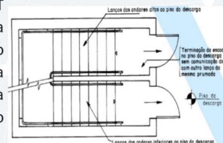
Figura 79: Escada enclausurada
