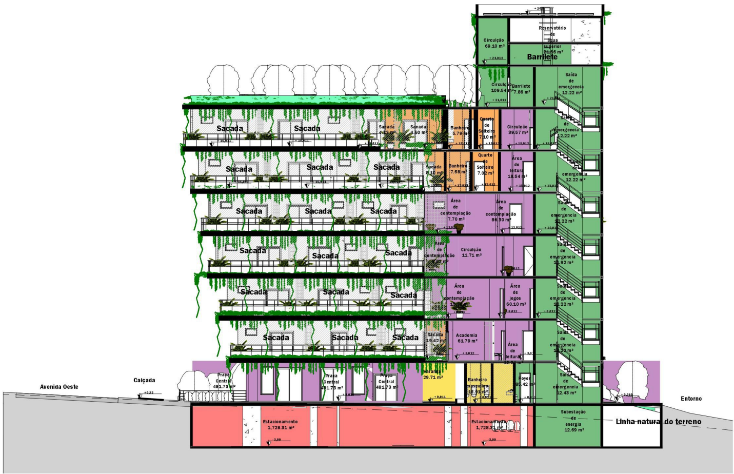
6.4.11.Corte BB
