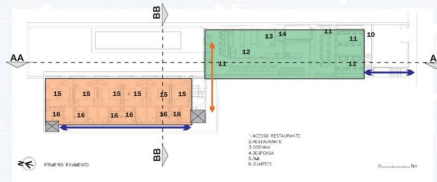
Figura 28: Planta primeiro pavimento setorizada. Fonte: ALVARENGA, MAIA e ZAMPIERI (2016). Edição: MORAIS, Rhayssa (2018).
