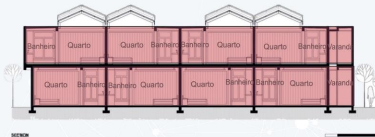
Figura 21: Corte BB setorizado Fonte: studiosaxe.com Edição: MORAIS, Rhayssa (2018)
