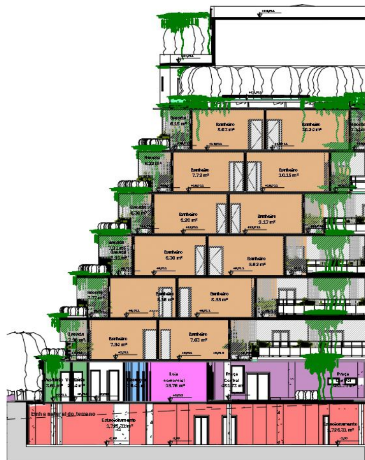
5.4.17.Corte HH Esc: 1/275
