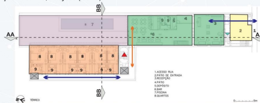
Figura 27: Planta térreo setorizada Fonte: (ALVARENGA, MAIA e ZAMPIERI (2016) Edição: MORAIS, Rhayssa (2018)
