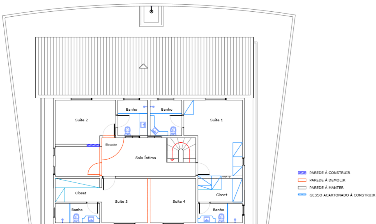
Figura 03: Planta baixa modificações pavimento térreo.
