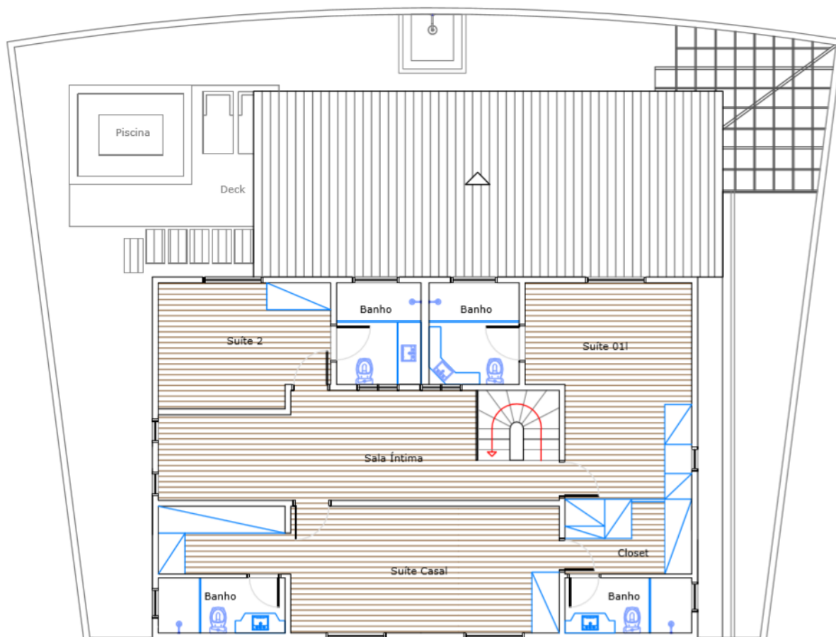
Figura 02: Planta baixa pavimento superior.
