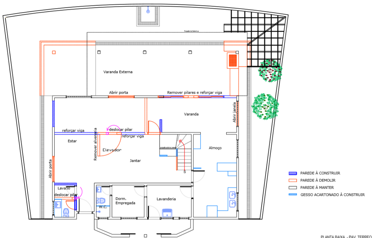
Figura 03: Planta baixa modificações pavimento térreo.
