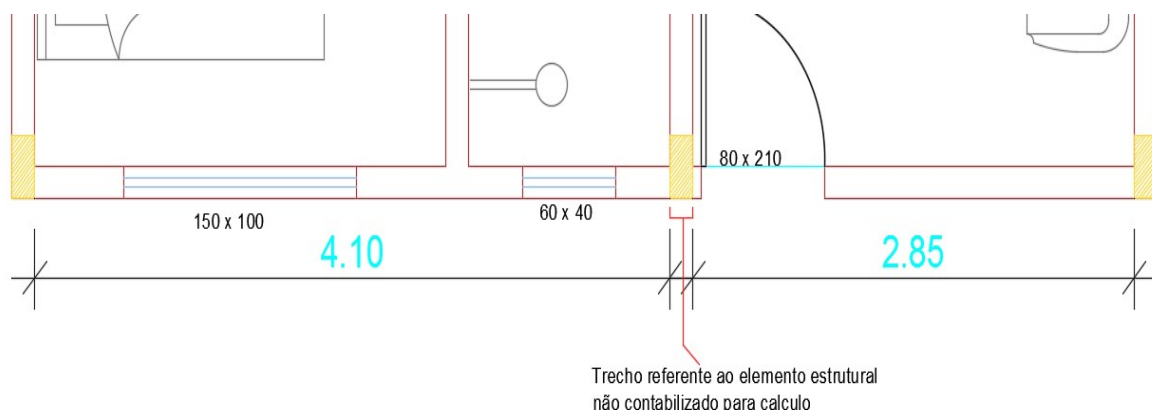
Figura 3. Cotas, descontando os trechos provenientes á estruturas.
