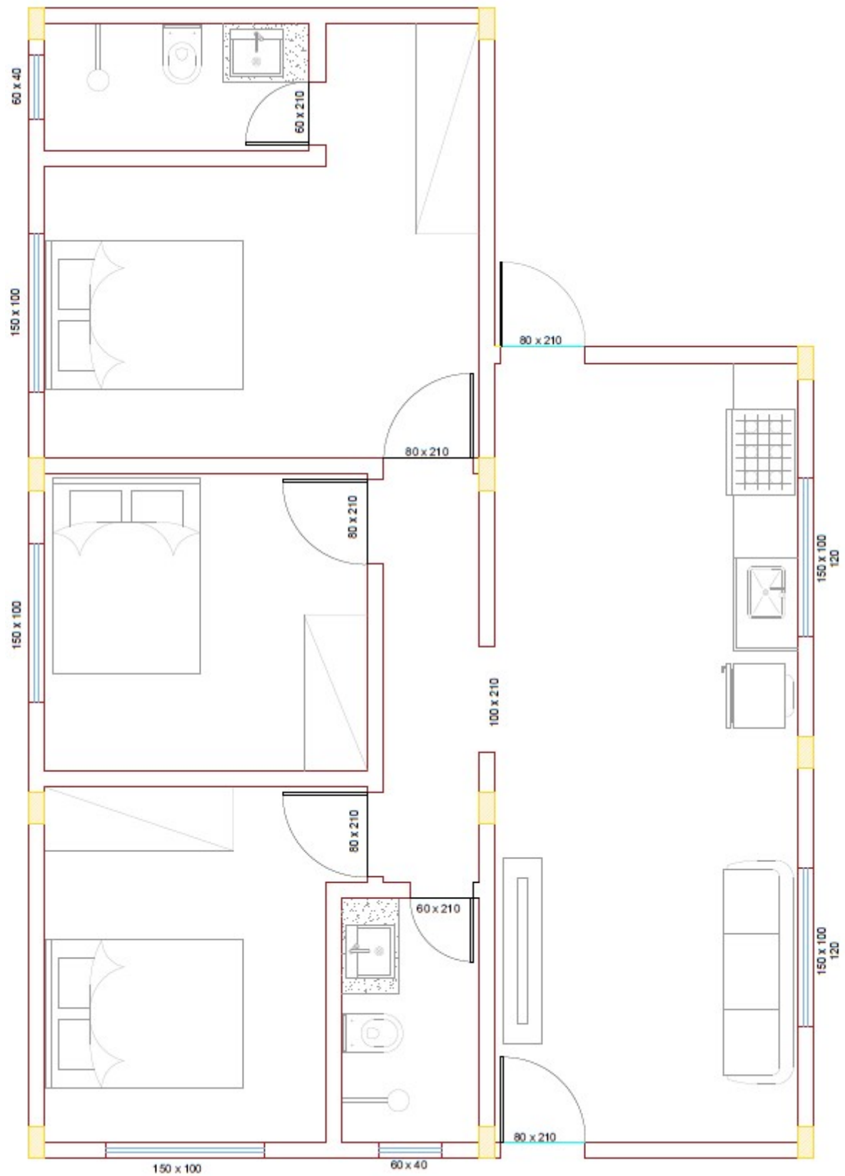
Figura 2. Planta Baixa com inserção de elementos estruturais (Pilares). Fonte: Imagem desenvolvida e retirada através do Software AutoCAD.
