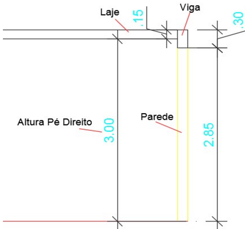
Figura 5. Representação da Altura da Alvenaria.
