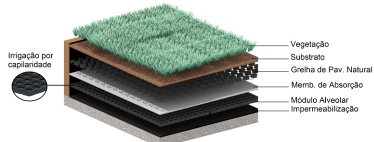
Telhado verde e suas camadas. Fonte: GoogleImagens
