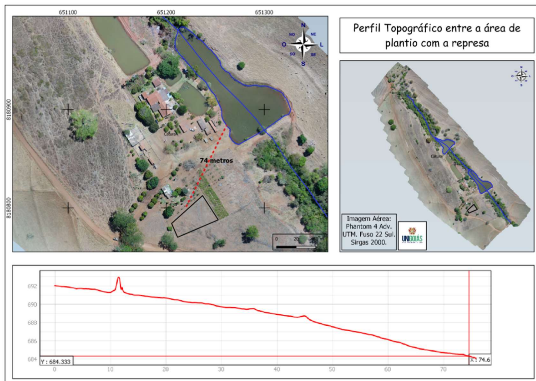
Figura 14. Perfil topográfico entre a área de plantio e a represa.
