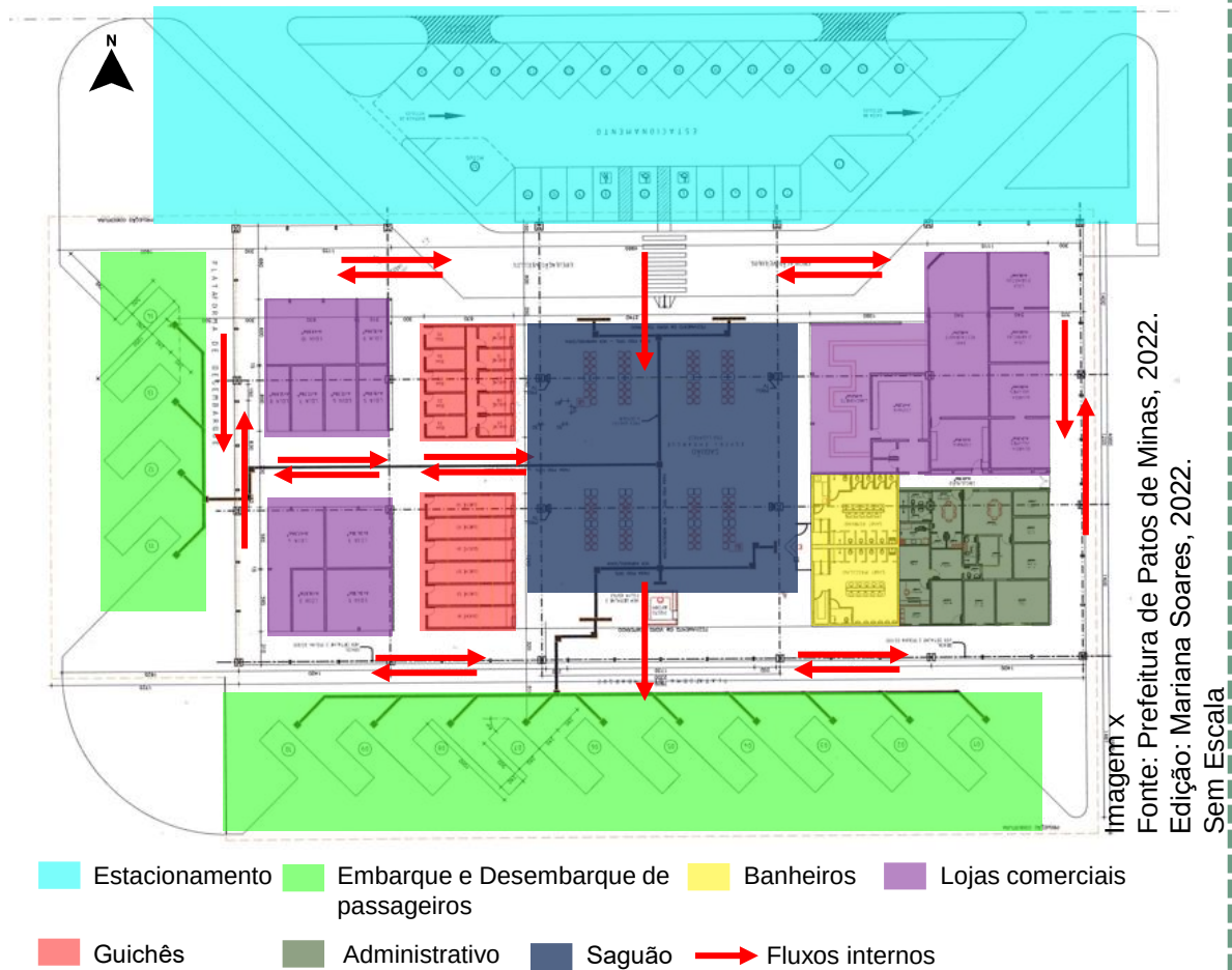
Planta Atual da Rodoviária
