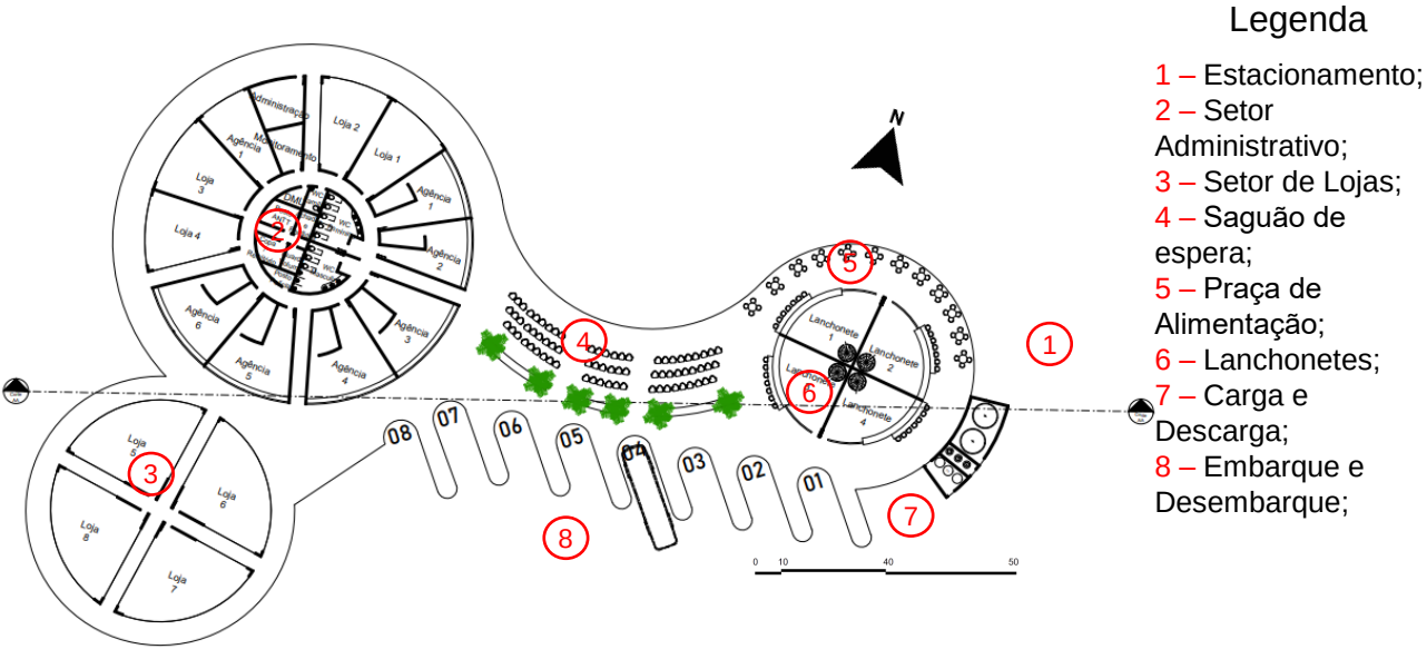
Planta Nova da Rodoviária
