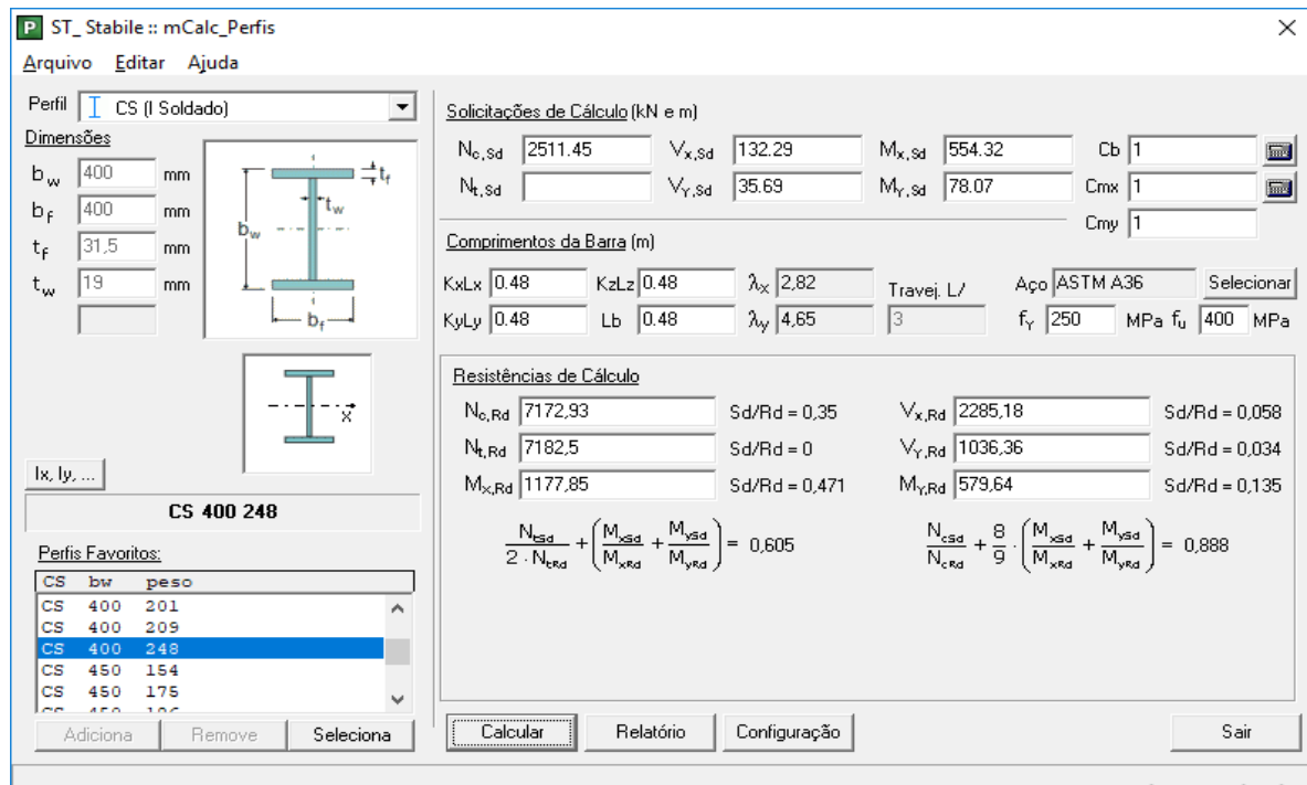
Figura 13. Dimensionamento dos pilares intermediários P11 e P14, adicionando a M_x e M_y seus respectivos momentos excêntricos, gerados por N_c a uma distância de 200mm do centro geométrico do pilar.
