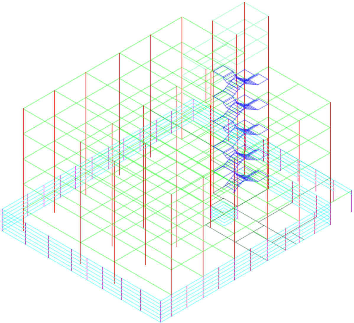
Figura 3. Modelo estrutural tridimensional. Fonte: Elaborado pelo próprio autor.
