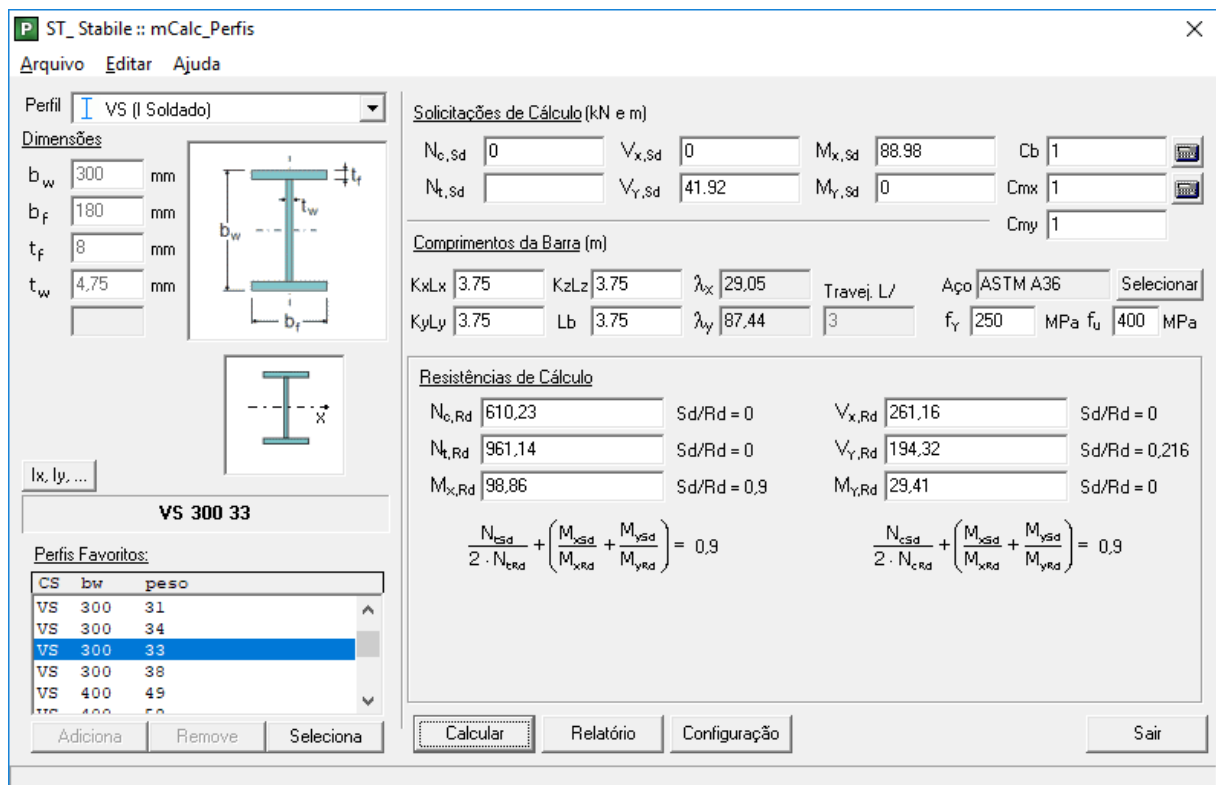
Figura 12. Dimensionamento da viga de aço VI14b, do pavimento térreo. Fonte: mCalcPerfis®.
