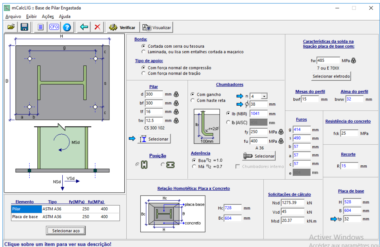
Figura 14. Dimensionamento da ligação da base de pilar engastada, P7 e P16. Fonte: mCalcLIG®.
