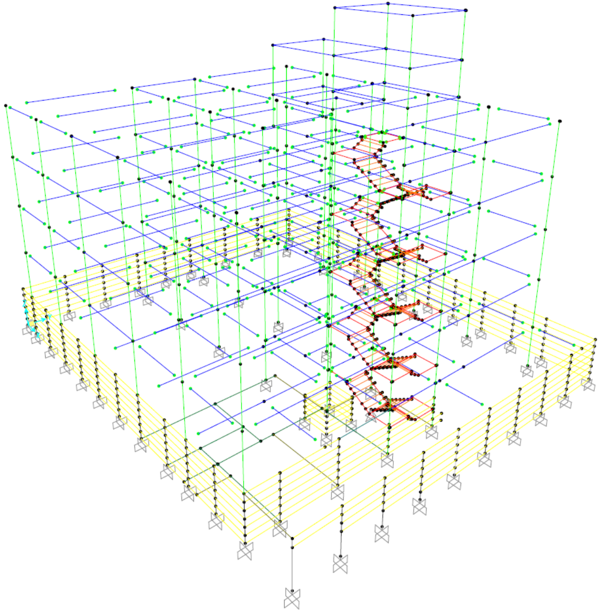
Figura 5. Estrutura pronta para receber os carregamentos. Fonte: SAP2000®.
