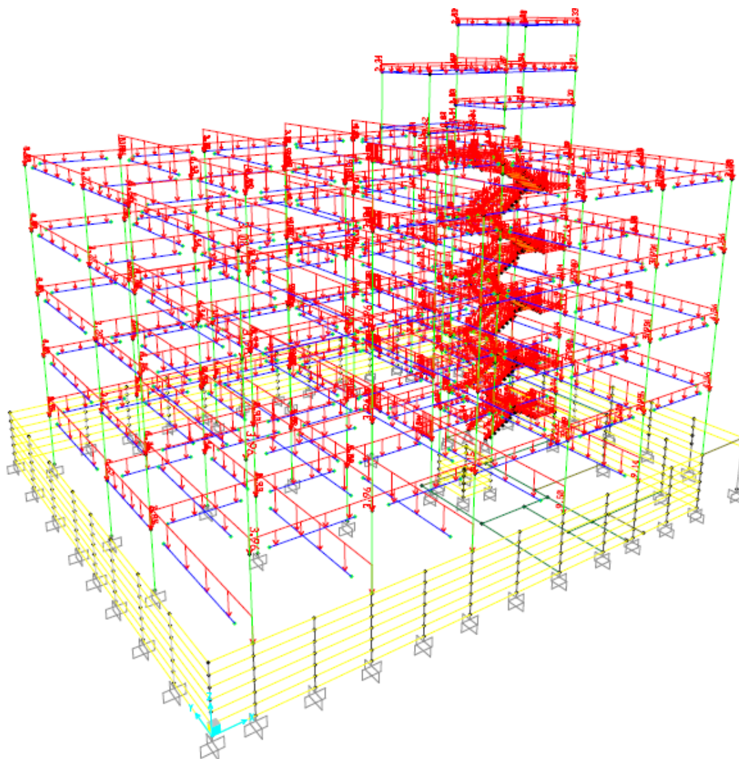
Figura 6. Estrutura carregada com o peso próprio da laje. Fonte: SAP2000®.
